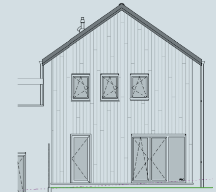
Pignon gauche
